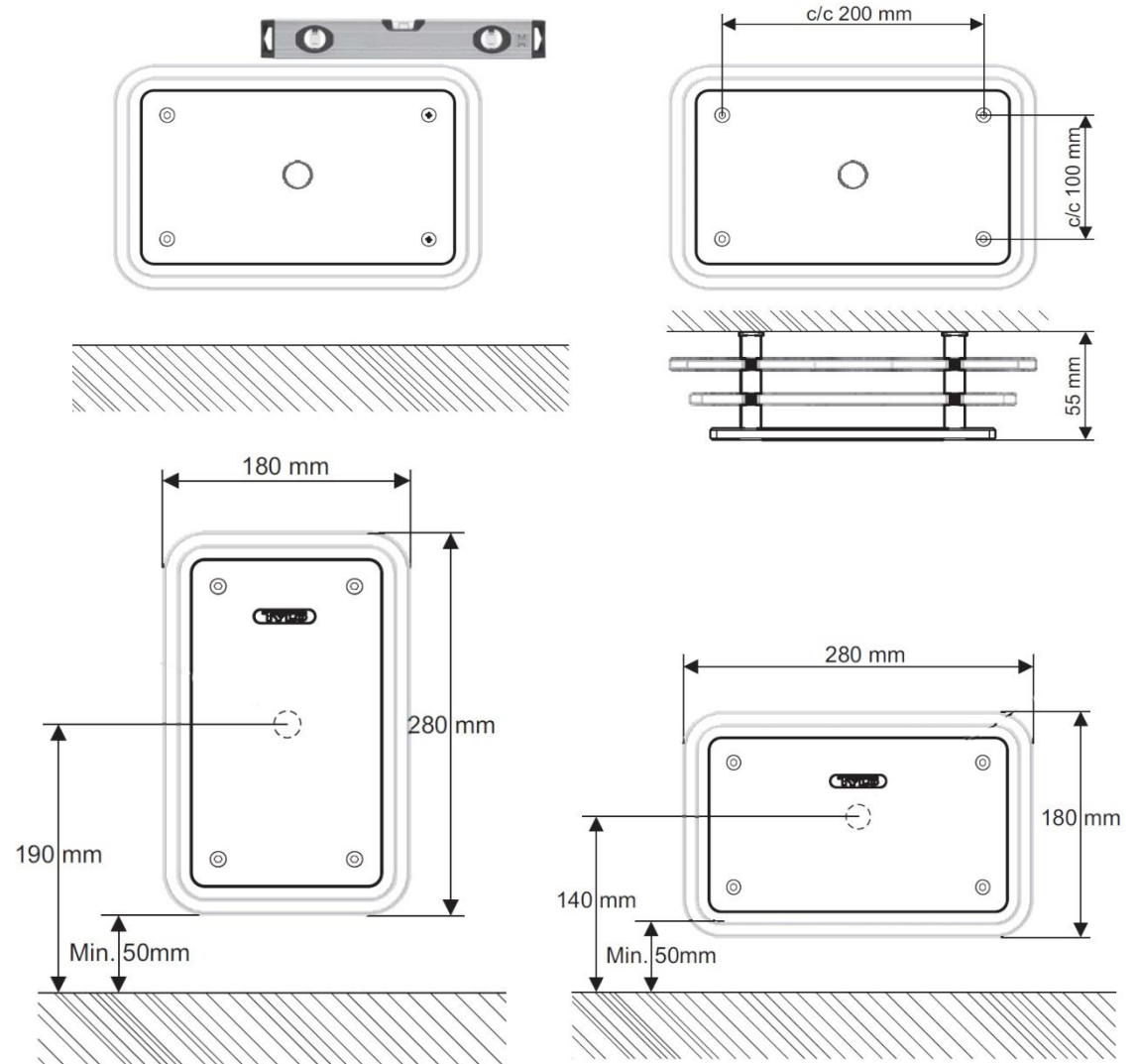
吹き出し口詳細図
